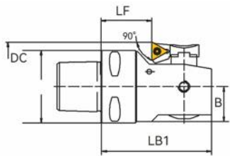
反镗
