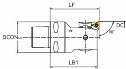
正镗
