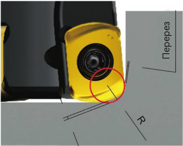
Технические данные программируемого радиуса R
